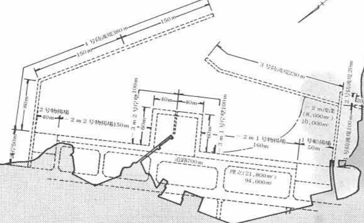
不知火海唯一の漁港となる平国港の計画図
